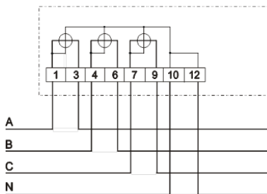
Рис.А.2 – Схема включения трехэлементного счетчика прямого включения в четырехпроводную сеть 0,4 кВ.
